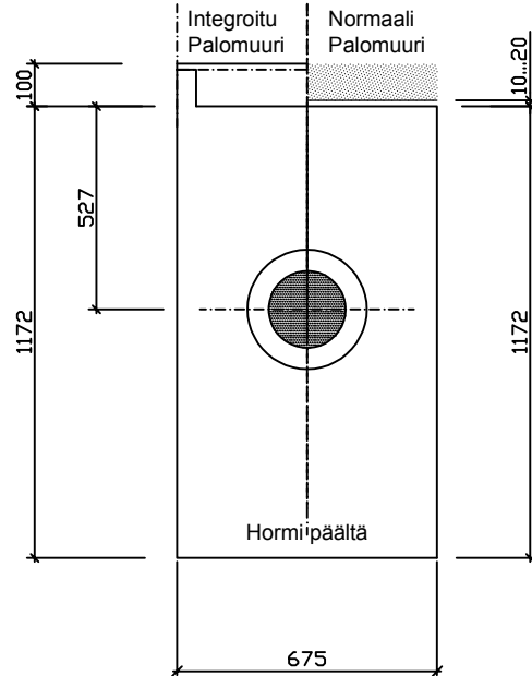
Mitat runkomittoja.
