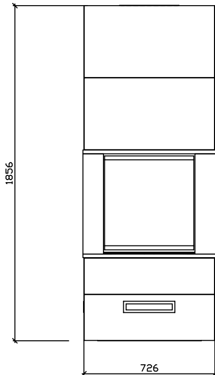
Mitat ulkomittoja.
