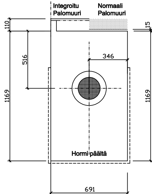
Mitat runkomittoja.
