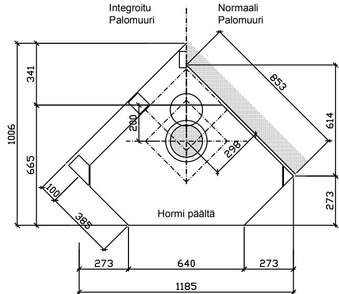
Mitat runkomittoja.
