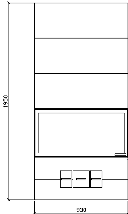
Mitat ulkomittoja.
