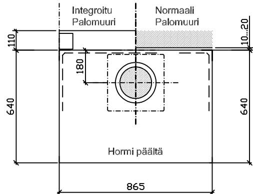
Mitat runkomittoja.
