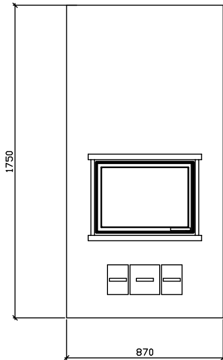
Mitat ulkomittoja.
