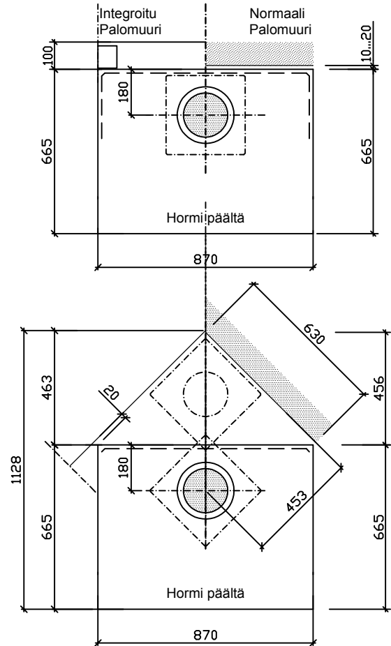
Mitat runkomittoja.
