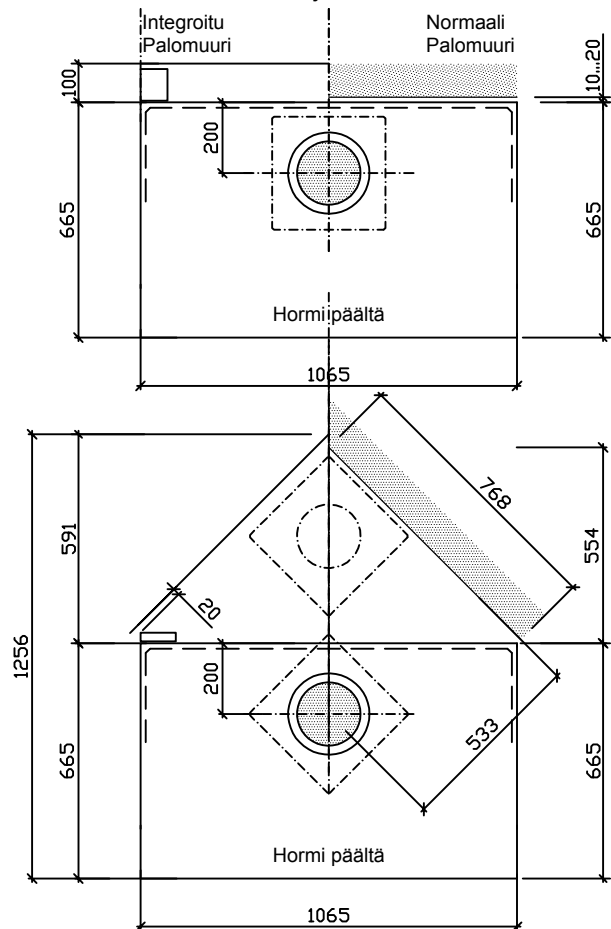
Mitat runkomittoja.
