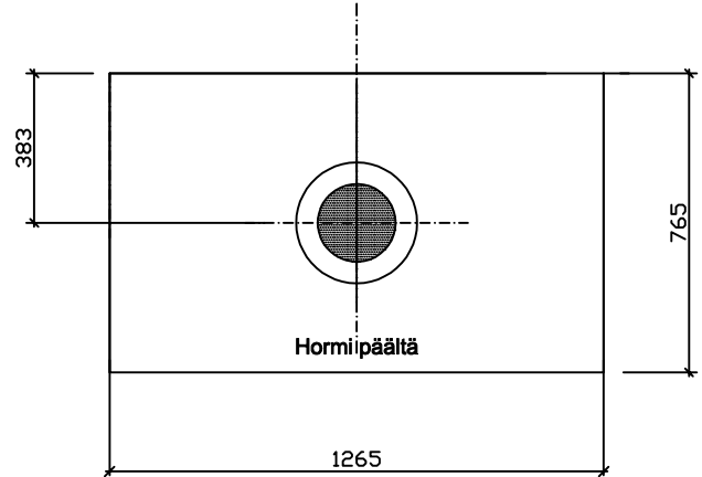
Mitat runkomittoja.
