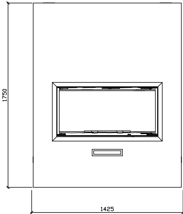
Mitat ulkomittoja.
