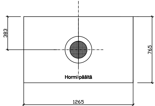
Mitat runkomittoja.
