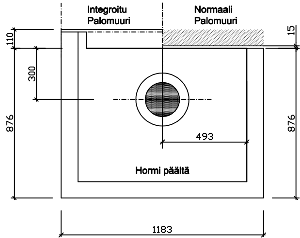
Mitat runkomittoja.
