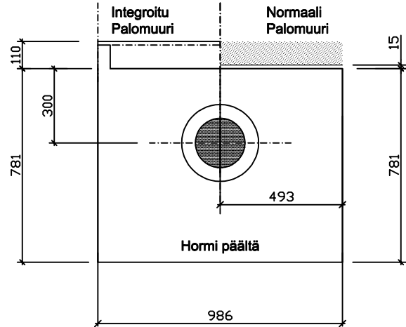
Mitat runkomittoja.
