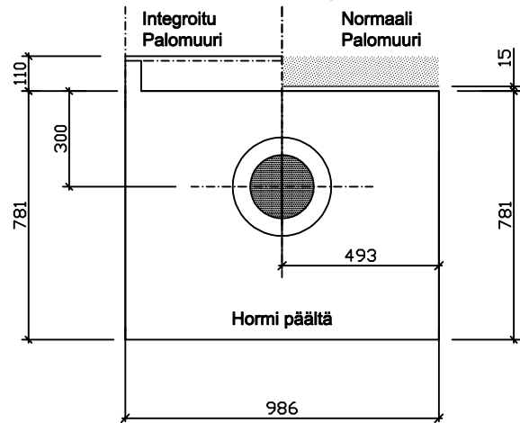
Mitat runkomittoja.
