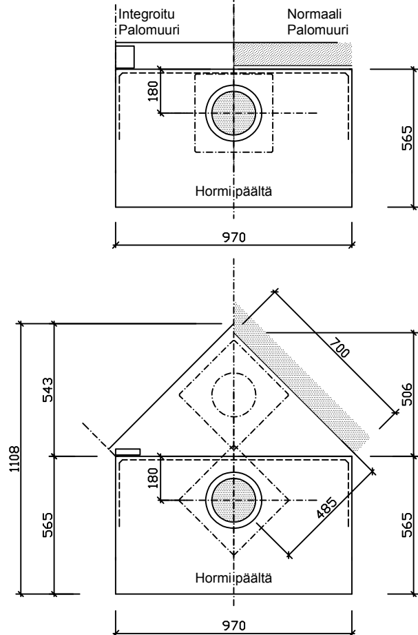
Mitat runkomitot.
