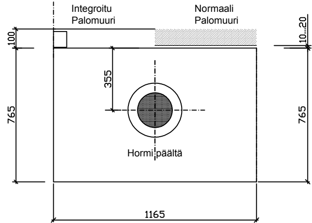
Mitat runkomittoja.
